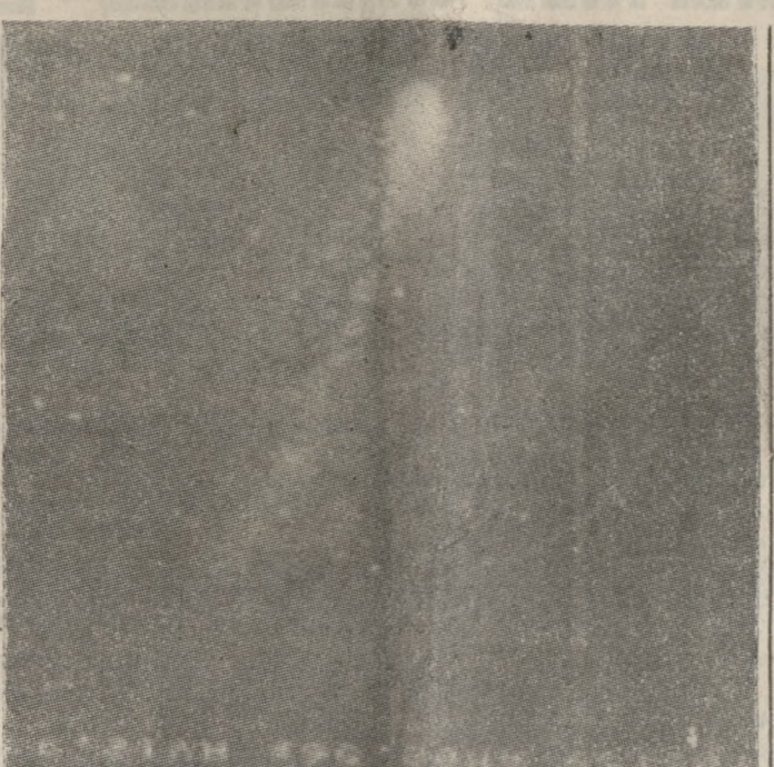
Μία από τις πρώτες φωτογραφίες του Κομητιού Χάλε' από το Αστεροσκοπείο του Σκίνακα. Το μέγεθος που η ούρα του Χάλε' καταλαμβάνει στον ουρανό είναι περίπου 1,5 μοίρες, δηλαδή 3 φορές περισσότερο το μέγεθος του φεγγαριού.
