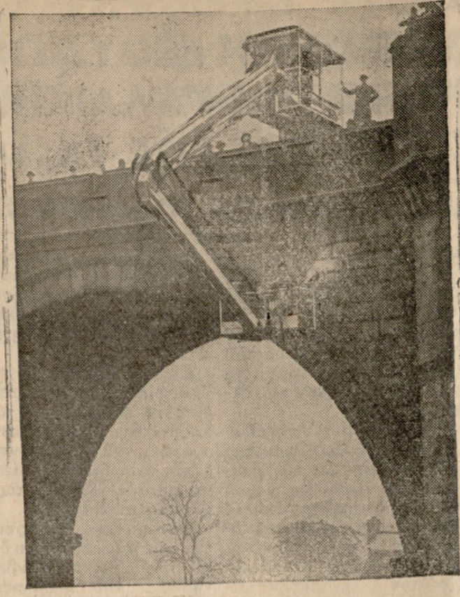
Η Έταιρεία Βρετανικών Σιδηροδρόμων κατασκεύασε και χρησιμοποιεί ένα μηχανήμα με το όποιον επιθεωρούνται εύκολα και γρήγορα αι γεφυροί. Τοποθετείται επάνω εις ένα μεγάλο σιδηροδρομικό βαγόνι και φθάνει μέχρι του κάτω τμήματος του τόξου μίας γεφύρας.
