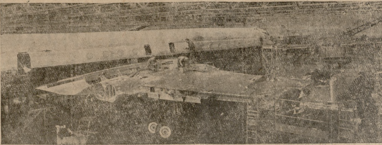
Μία φωτογραφία από την συναρμολόγησιν αεροσφαιρούμενων επίβατικών αεροπλάνων «Κομήτης 4 Β» διά λογαριασμόν της Έλληνικής Εταιρείας «Ολυμπιακή αεροπορία».
