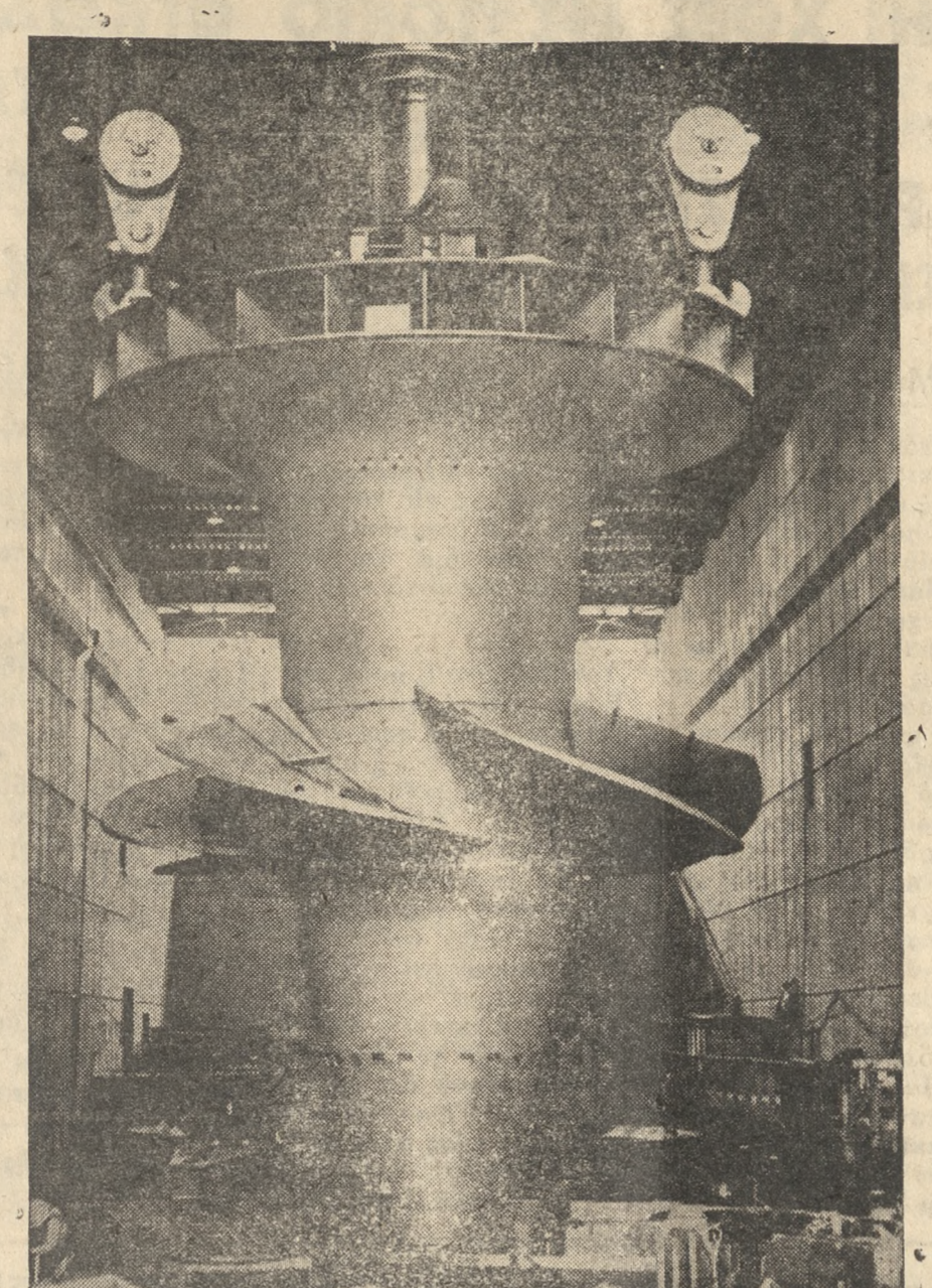
Ὁ ἄνω στρόβιλος Βρετανικῶς τοποθετεῖται εἰς ἕνα ὑδροηλεκτρικὸν σταθμὸν πλησίον τῆς Οὐάσιγκτον καὶ ἀποτελεῖ μέρος μίας παραγωγικῆς ὑδροστρωβίλων δυνάμεως 114.000 ἵππων καὶ ἐξετάσθησαν Βρετανικὴ ἑταιρεία διὰ τὰς Ἠνωμένας Πολιτείας.
