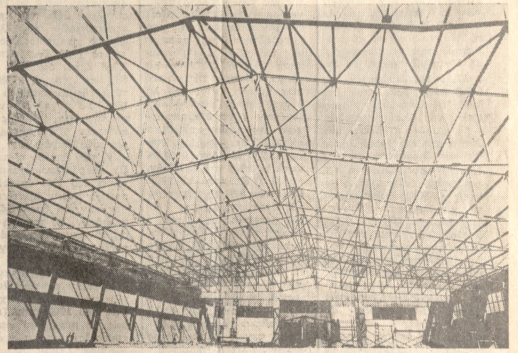
Στέγη από δομικόν μορφοσίτηρον του κτιρίου των Γενικών Άποθηκών εις Πειραιά, κατασκευασθείσα από τον Κλάδον Σιδηρών Κατασκευών της Ντέξιον Έλλάς Α.Ε. Εις την δραστηριότητά του Κλάδου αυτού της Ντέξιον έδεν να καταλογισθή ή πραγματοποίησις έκτετατών μέχρι τούδε μεγάλων κατασκευών, έπως στεγών και έκκεληρων σκελετών έργαστασιών, γεφυρών, γερανογεφυρών του ΝΑΤΟ, γκαράζ μεγάλων άνοιγμάτων, κλειστών Γυμναστηρίων, έσχατών ύβρεληφίσις και καλύμματα γεννητριών δια φράγματι της ΔΕΗ, πυλώνων κλπ.
