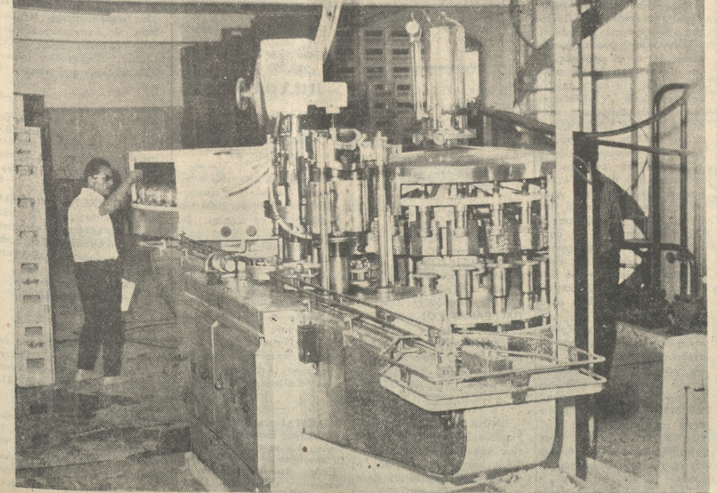
Τὸ αὐτόματο μηχανήμα ἐμφιαλώσεως καὶ πωματισμοῦ.
