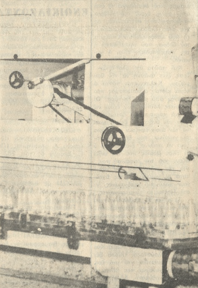
Τὸ αὐτόματο μηχανήμα πλῶσεως καὶ ἀποστειρώσεως τῶν φιαλῶν.
