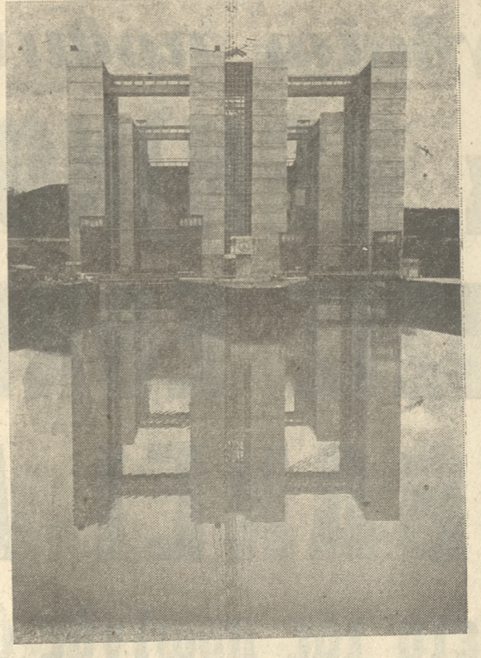
Λέμβοι — Οἰρώγια, βάρος 1.350 τόνων. Τὸ ὠφέλιμον μήκος τῶν κολυμάτων (σκάφες) πού λειτουργοῦν ἀνεξάρτητα μεταξύ τῶν ἀνέρχεται εἰς ἑκατὸ μέτρα τὸ κράτος εἰς δώδεκα μέτρα εἰς δὲ πλῆρη μετ' ὕδωρ εἰς ὕψος 3,5 μέτρων. Τὰ κολυμματα αὐτὰ ἐκ χάλυβος βάρους 5.700 τόνων θὰ λειτουργοῦν ἐξ ἄλλου συμφῶνως πρὸς τὸ ἀξίωμα τῶν ἀνελευστηρίων ἀτέρμονος ἀλυσῶν (πατερνώστερ).
