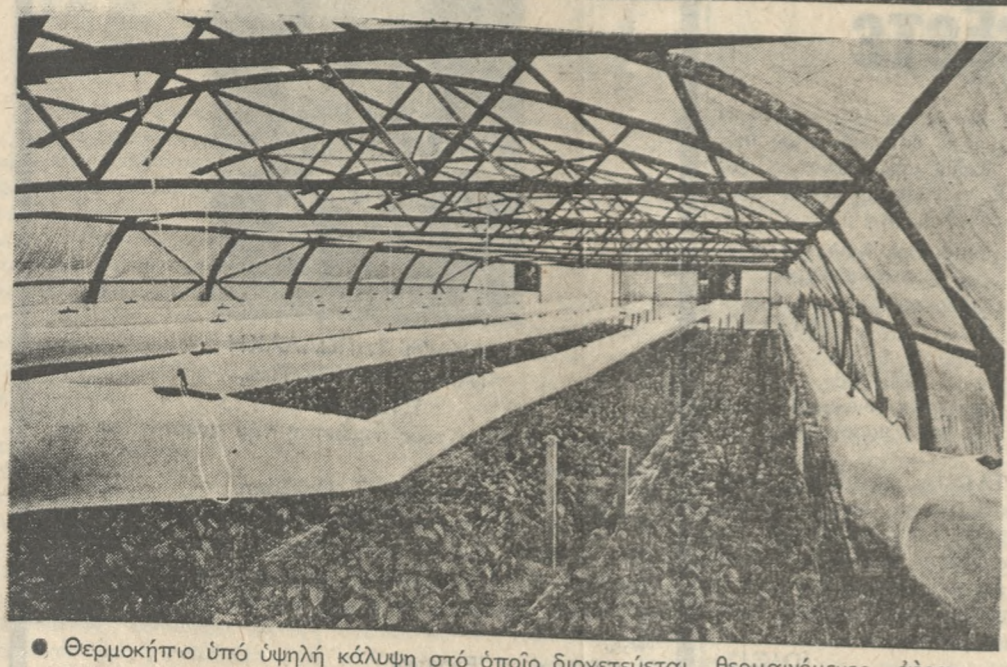
Θερμοκήπιο υπό υψηλή κάλυψη στο οποίο διαχεύεται θερμαινόμενος αέρας μέσω πλαστικών σωλήνων.
