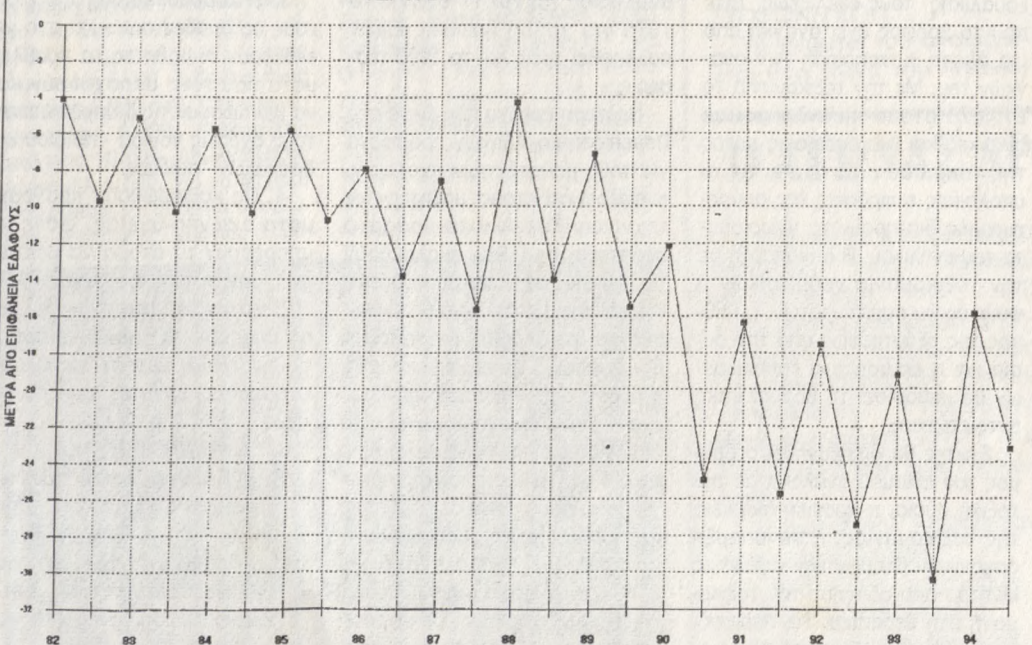
ΔΙΑΓΡΑΜΜΑ ΔΙΑΚΥΜΑΝΣΗΣ ΣΤΑΘΜΗΣ ΥΔΡΟΓΕΩΛΟΓΙΚΗ ΛΕΚΑΝΗ ΒΙΑΝΝΟΥ
